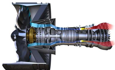
도표 281. GTF(Geared Turbofan) 엔진
