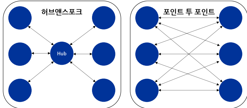
도표 101. 허브앤스포크와 포인트 투 포인트 개념도
