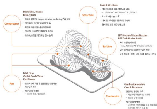
도표 275. 한화에어로스페이스 주요 엔진 부품
