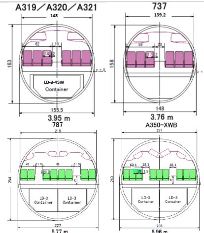
도표 155. 협동체와 광동체 비교
