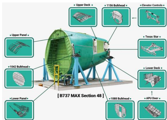
도표 307. 대표 제품 B737 Section 48
