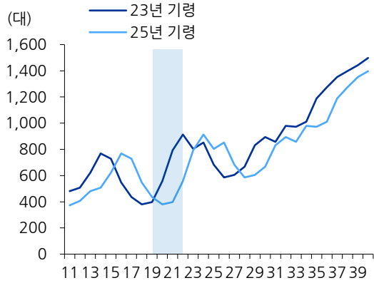
도표 147. 항공기 퇴역 추정
