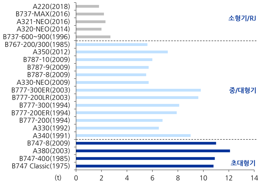
도표 136. 1 LTO 사이클 당 이산화탄소 배출량
