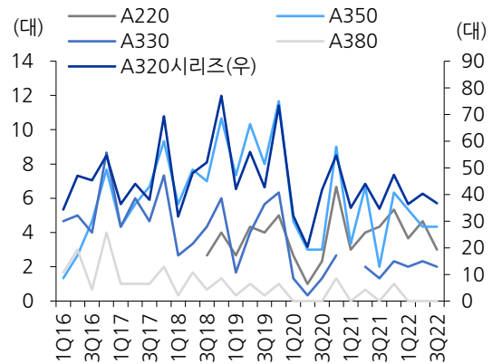
도표 170. 에어버스기종별 월간 생산대수
