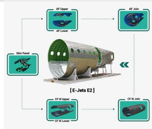
도표 316. 아스트 공급 부품(중/후방 동체)
