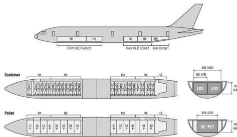
도표 70. 벨리 카고 개요
